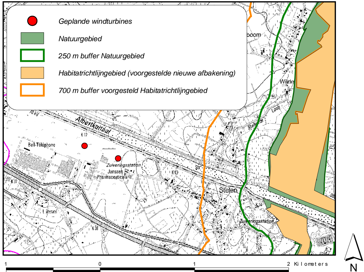
Figuur 1: Inplantingsplaats van 2 geplande windturbines, met aanduiding van Natuurgebied en voorgesteld Habitatrichtlijngebied (annex 250 en 700 m buffers).
