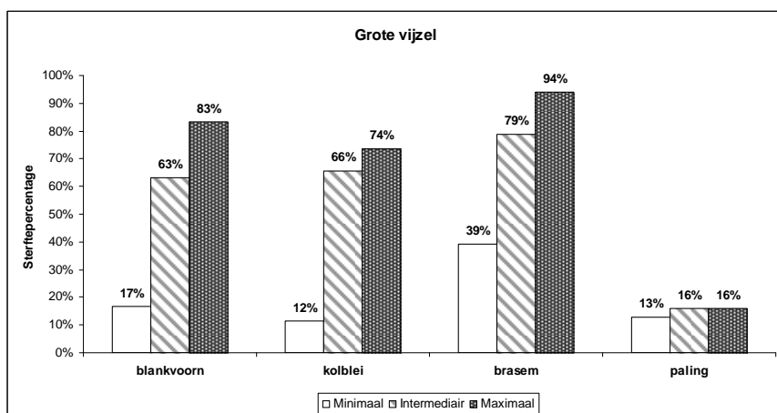
Figuur 21: Sterftepercentages berekend volgens de verschillende scenario's voor de vier dominante vissoorten die de grote vijzel passeerden.
