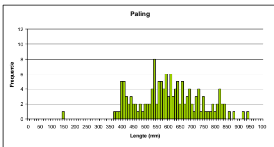
Figuur 13: Lengtefrequentieverdeling van de gevangen paling.
